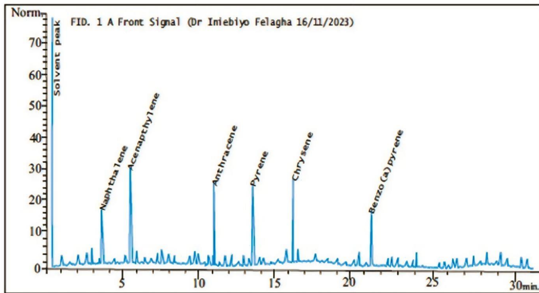
Fig. 1. GC-FID chromatogram of Achi (Brachystegia eurycoma)
